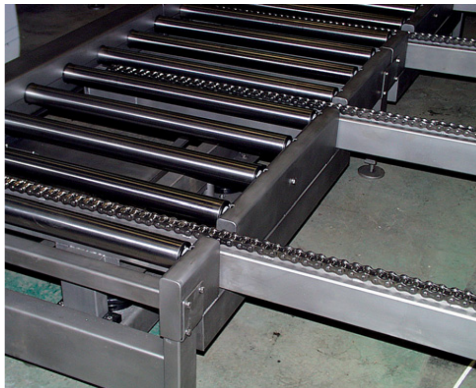
Rustfrit transportanlæg bestående af rullebaner med integreret kædebaner for løft og sideudtræk. Leveret til Chr. Hansen A/S.
